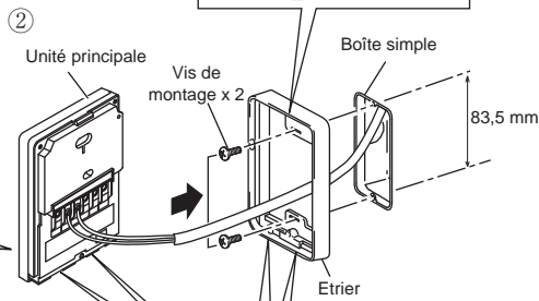
Face avant
