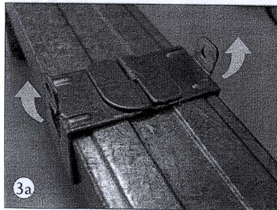
3a Per il fissaggio alle staffe piegare le due alette
