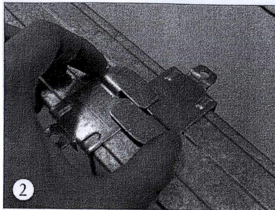
2 Innestare tra di loro le due staffe. Eventualmente aiutarsi con una pinza.
