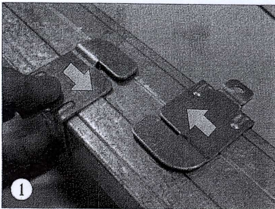
1 Posizionare le due staffe sulla guida
