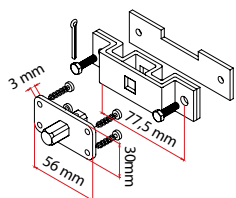
Kit support patte entreaxe 77,5 mm et axe carré 10 mm
