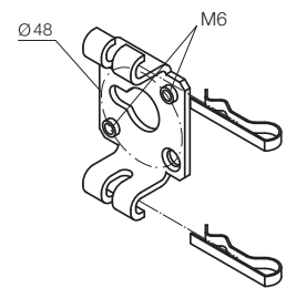
525.10051 max 80 Nm Support standard avec 2 trous filetés M6
