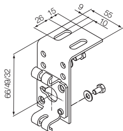
525.10053 max 80 Nm Support standard sur bride réglable sur 3 positions
