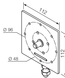
525.10047 Bride réglable avec Ø 10 mm
