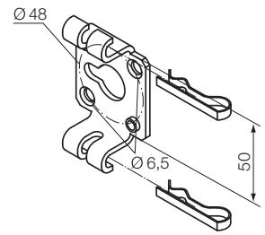
525.10040 max 80 Nm Support standard avec 2 trous fraisés Ø 6,5 mm
