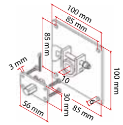
Kit support plaque 100x100 avec déverrouillage et axe carré 10 mm
