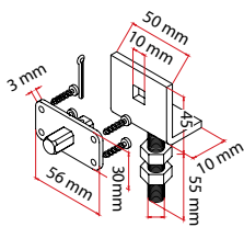
Kit support patte réglable et axe carré 10 mm
