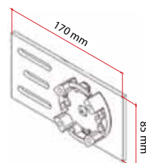
Support monobloc côté moteur
