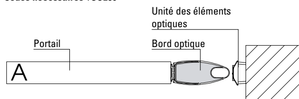
Fig. B - Sur profilé contre-butée
