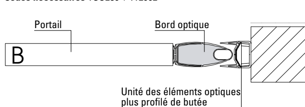
Fig. B - Sur profilé contre-butée
