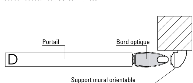
Fig. D - Sur support mural à orientation réglable
