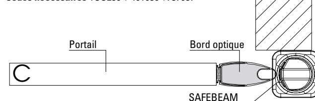
Fig. D - Sur support mural à orientation réglable
