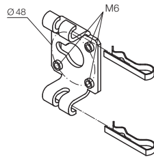
525.10067 max 80 Nm Support standard avec 4 trous filetés M6
