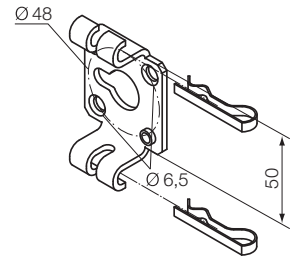
525.10040 max 80 Nm Support standard avec 2 trous fraisés Ø 6,5 mm
