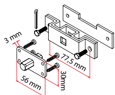
Kit support patte entraxe 77,5 mm et axe carré 10 mm
