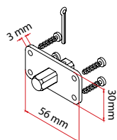
Support Axe carré 10 mm
