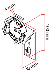
Support avec dépassement 40 mm
