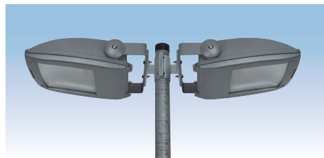
Montage avec deux supports pour mât
