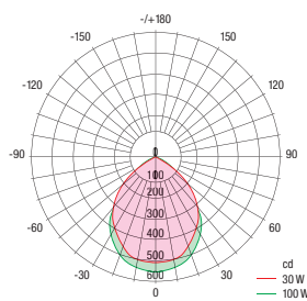
Projecteur LED 30W et 100W
