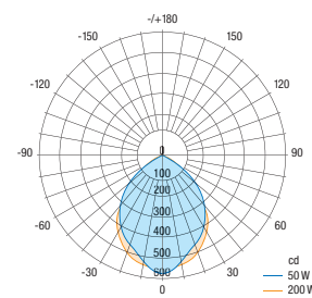
Projecteur LED 50W et 200W
